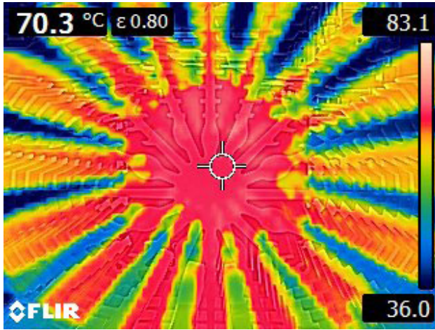
ARMAGEDDON® ile Isı Dağılımı
