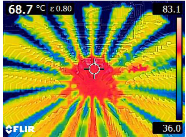
Geleneksel Yöntemde Isı Dağılımı
